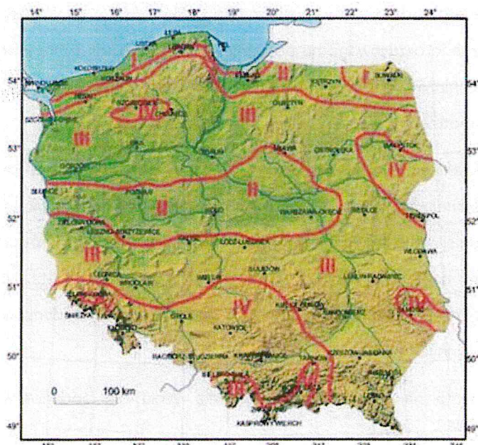
Rysunek 9. Strefy energetyczne wiatru w Polsce. Źródło: Baza Danych Odnawialnych Źródeł Energii.
